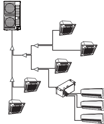
✧ Using Y-joint Using Y-joint / EEV kit
